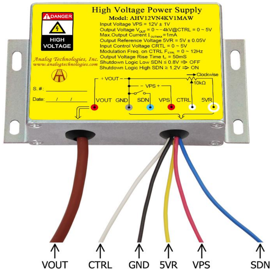
图 1、AHV12VN4KV1MAW 俯视图
