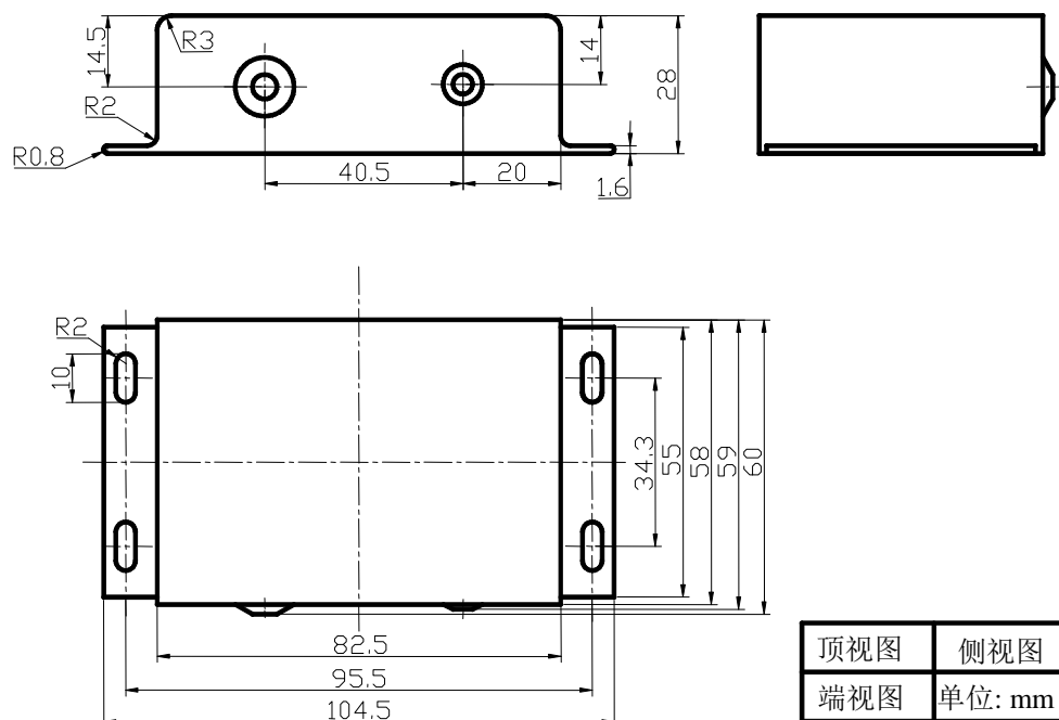
图12、AHV12VN4KV1MAW的尺寸
