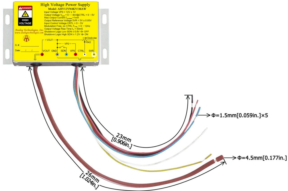
图11、AHV12VN4KV1MAW的导线
