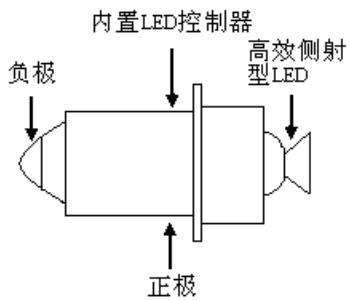
图 3. SILVERLED-1N6V 的侧视图
