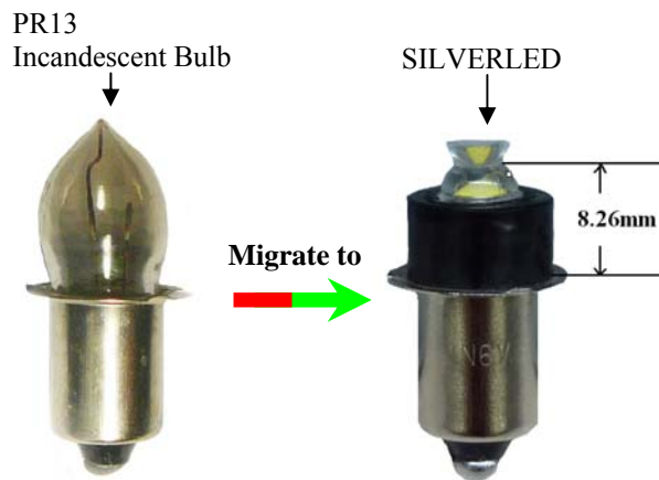
图 2. 白炽灯泡被 SILVERLED 所替代
